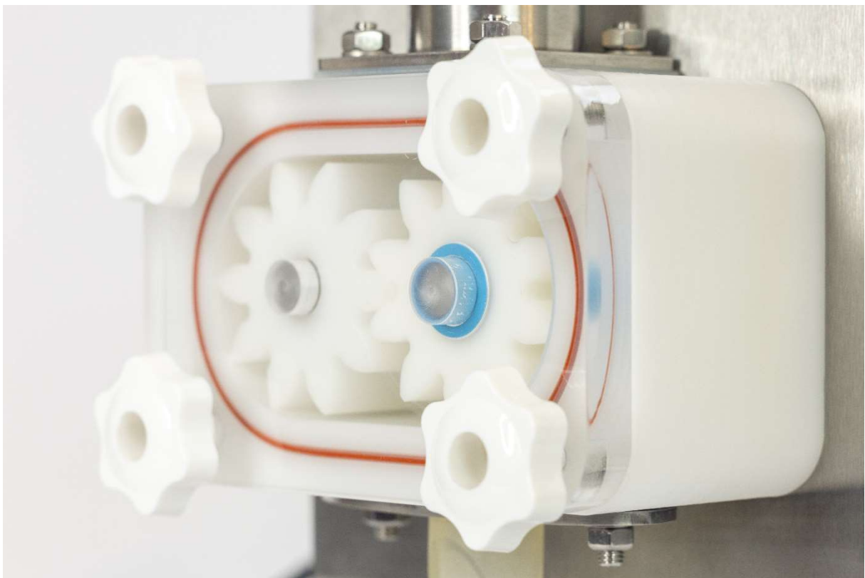
Pumpenkopf mit integrierten Zahnradern
